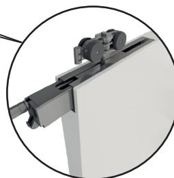
UCHWYT REGULOWANY - OPCJONALNIE ADJUSTABLE HANGER - AS OPTION
